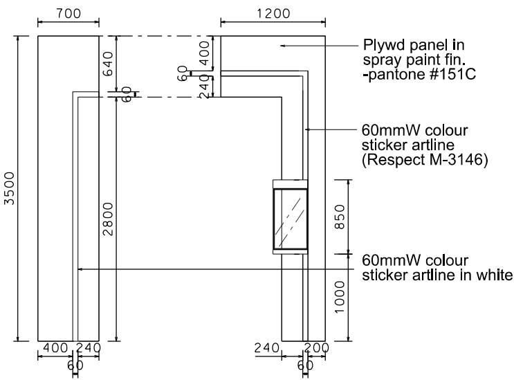
FACSCIA ELEVATION
